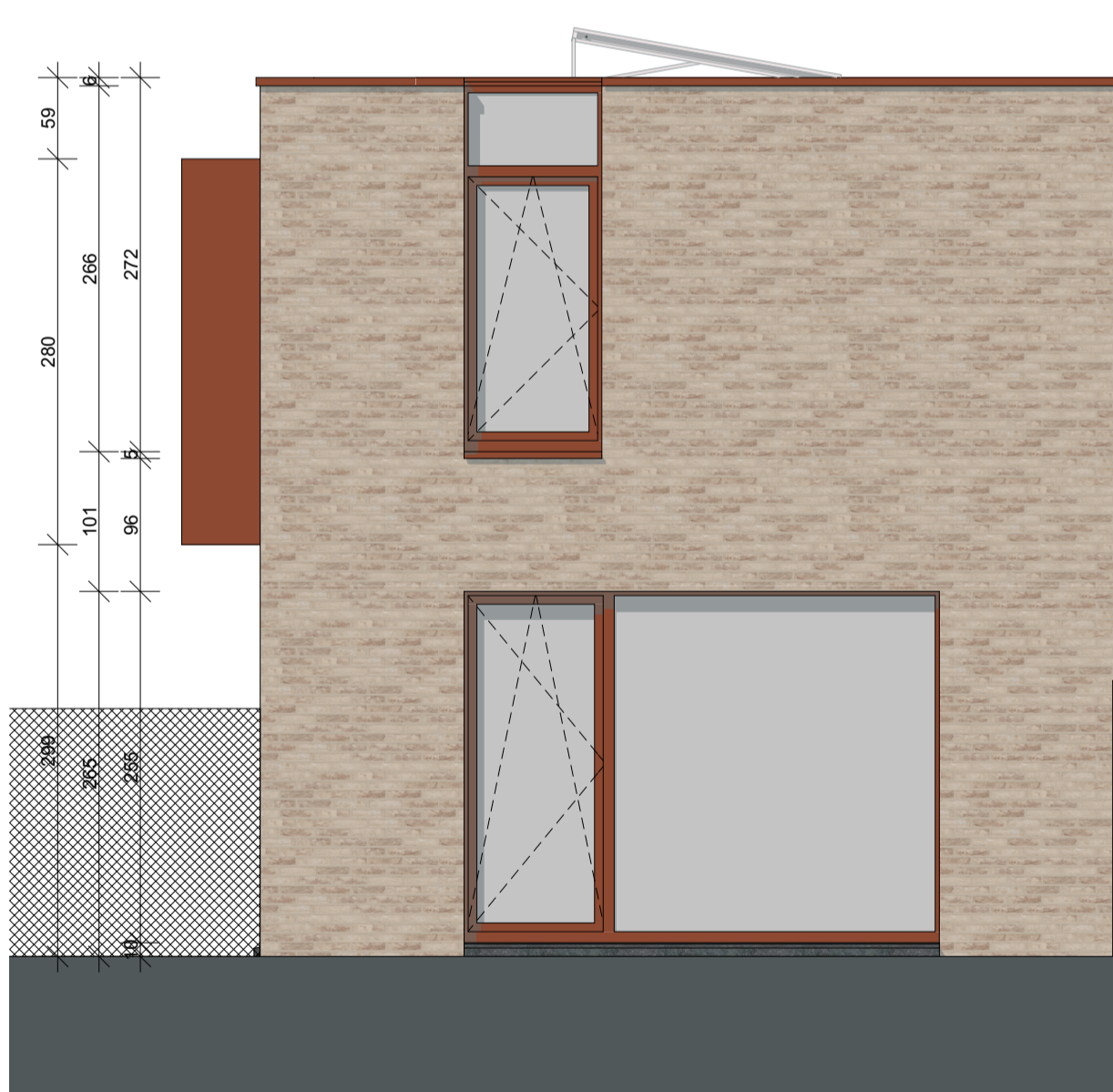
Achtergevel
