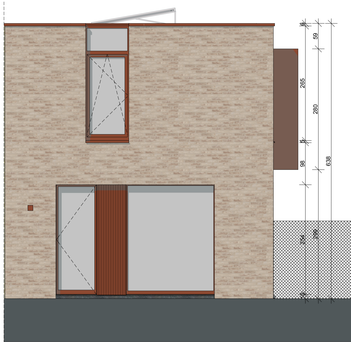
Voorgevel
