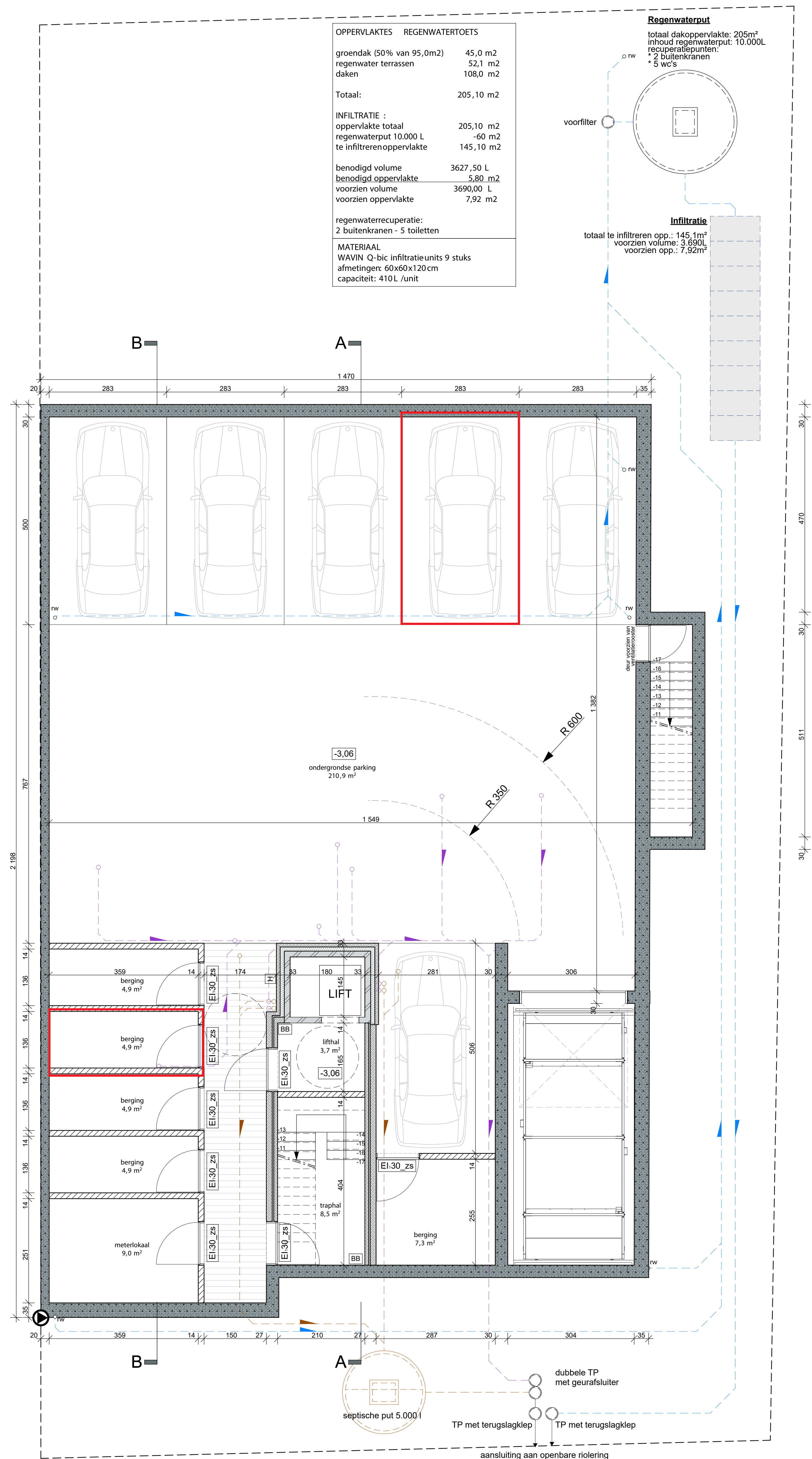
funderings- en rioleringsplan
