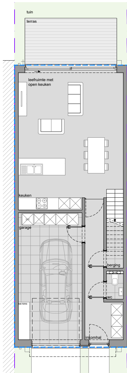
Gelijkvloers
