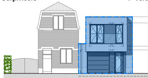
Voorgevel
