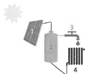
1. Zonnecollector | 2. Opslagvat warmwater | 3. Sanitair warm water | 4. Aankoppeling aan ruimteverwarming (radiator)
